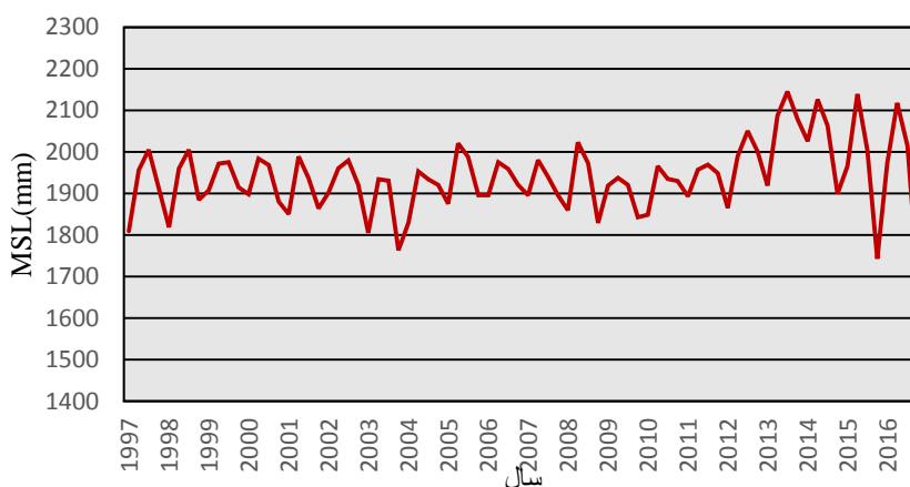
شکل ۲- روند تغییرات سالانه‌ی میانگین تراز آب دریا در ایستگاه جاسک
