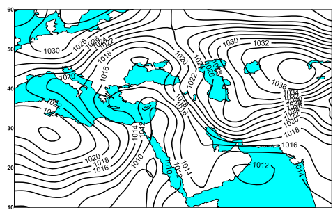
شکل ۱۵- میدان فشار (hpa) در ساعت ۰۰۰۰ گرینویچ ۱۲ مارس ۲۰۱۵.
