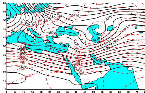
شکل ۳۳- میدان ارتفاع ژئوپتانسیل (gpm) و دما (k) در تراز ۵۰۰ هکتوپاسکال در ساعت ۰۰۰۰ گرینویچ ۱۷ ژانویه ۲۰۰۰.
