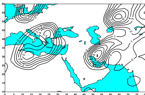
شکل ۲۳- میدان تاوایی در تراز ۵۰۰ هکتوپاسکال در ساعت ۰۰۰۰ گرینویچ ۱۱ مارس ۲۰۱۵.
