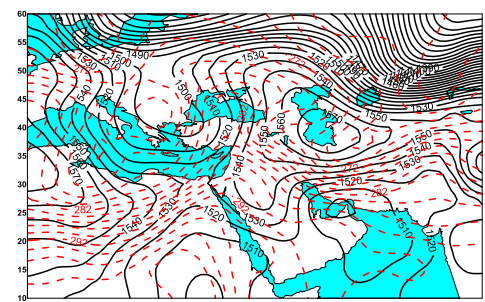
شکل ۸- میدان ارتفاع ژئوپتانسیل (gpm) و دما (k) در تراز ۸۵۰ هکتوپاسکال در ساعت ۰۰۰۰ گریجوی ۱۱ مارس ۲۰۱۵.
