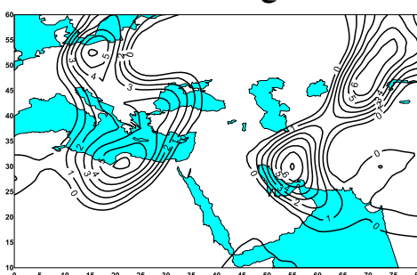
شکل ۲۵- میدان تاوایی در تراز ۵۰۰ هکتوپاسکال در ساعت ۱۲۰۰ گرینویچ ۱۱ مارس ۲۰۱۵.
