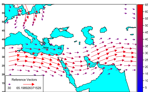
شکل ۳۴- میدان باد (m/s) در تراز ۲۰۰ هکتوپاسکال ساعت ۰۰۰۰ گرینویچ ۱۷ ژانویه ۲۰۰۰.
