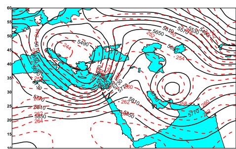
شکل ۱۷- میدان ارتفاع ژئوپتانسیل (gpm) و دما (k) در تراز ۵۰۰ هکتوپاسکال در ساعت ۰۰۰۰ گرینویچ ۱۲ مارس ۲۰۱۵.
