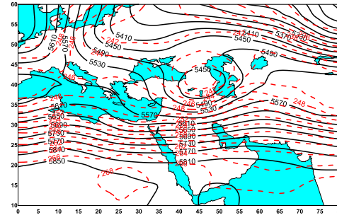
شکل ۳۱- میدان ارتفاع ژئوپتانسیل (gpm) و دما (k) در تراز ۵۰۰ هکتوپاسکال در ساعت ۰۰:۰۰ گرینویچ ۱۶ ژانویه ۲۰۰۰.
