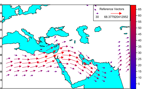
شکل ۱۸- میدان باد (m/s) در تراز ۲۰۰ هکتوپاسکال ساعت ۰۰۰۰ گرینویچ ۱۲ مارس ۲۰۱۵
