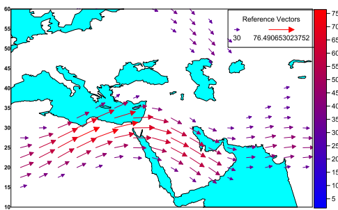
شکل ۶- میدان باد (m/s) در تراز ۲۰۰ هکتوپاسکال ساعت ۱۲۰۰ گریجوی ۱۰ مارس ۲۰۱۵
