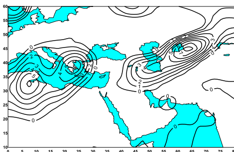
شکل ۲۱- میدان تاوایی در تراز ۵۰۰ هکتوپاسکال در ساعت ۰۰۰۰ گرینویچ ۱۰ مارس ۲۰۱۵. شکل ۲۲- میدان تاوایی در تراز ۷۰۰ هکتوپاسکال در ساعت ۰۰۰۰ گرینویچ ۱۰ مارس ۲۰۱۵.
