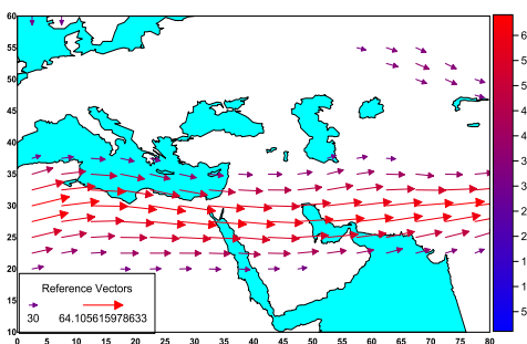
شکل ۳۰- میدان باد (m/s) در تراز ۲۰۰ هکتوپاسکال ساعت ۰۰:۰۰ گرینویچ ۱۶ ژانویه ۲۰۰۰.
