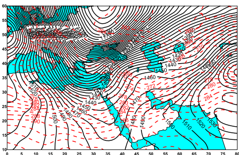
شکل ۳۶- میدان ارتفاع ژئوپتانسیل (gpm) و دما (k) در تراز ۸۵۰ هکتوپاسکال در ساعت ۰۰۰۰ گرینویچ ۱۸ ژانویه ۲۰۰۰.
