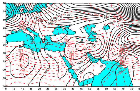
شکل ۲۸- میدان ارتفاع ژئوپتانسیل (gpm) و دما (k) در تراز ۸۵۰ هکتوپاسکال در ساعت ۰۰:۰۰ گرینویچ ۱۶ ژانویه ۲۰۰۰.
