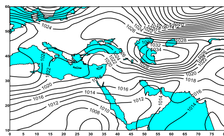
شکل ۳- میدان فشار (hpa) در ساعت ۱۲۰۰ گرینویچ ۱۰ مارس ۲۰۱۵.
