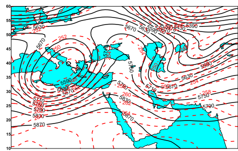
شکل ۵- میدان ارتفاع ژئوپتانسیل (gpm) و دما (k) در تراز ۵۰۰ هکتوپاسکال در ساعت ۱۲۰۰ گریجوی ۱۰ مارس ۲۰۱۵.
