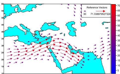
شکل ۱۰- میدان باد (m/s) در تراز ۲۰۰ هکتوپاسکال ساعت ۰۰۰۰ گریجوی ۱۱ مارس ۲۰۱۵
