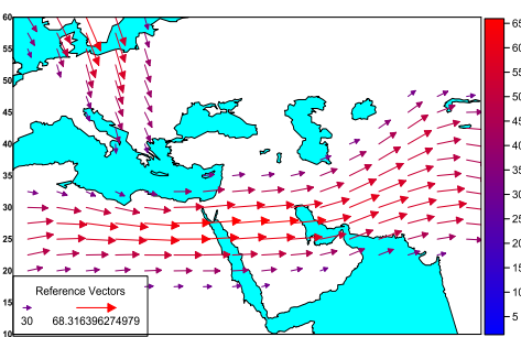
شکل ۳۸- میدان باد (m/s) در تراز ۲۰۰ هکتوپاسکال ساعت ۰۰۰۰ گرینویچ ۱۸ ژانویه ۲۰۰۰.
