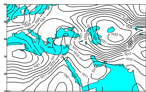
شکل ۱۱- میدان فشار (hpa) در ساعت ۱۲۰۰ گریجوی ۱۱ مارس ۲۰۱۵.
