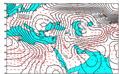
شکل ۱۲- میدان ارتفاع ژئوپتانسیل (gpm) و دما (k) در تراز ۸۵۰ هکتوپاسکال در ساعت ۱۲۰۰ گریجوی ۱۱ مارس ۲۰۱۵.
