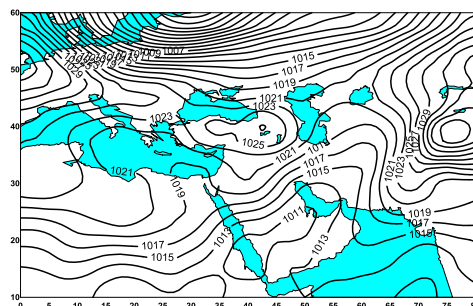
شکل ۳۱- میدان فشار (hpa) در ساعت ۰۰۰۰ گرینویچ ۱۷ ژانویه ۲۰۰۰.
