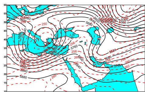
شکل ۹- میدان ارتفاع ژئوپتانسیل (gpm) و دما (k) در تراز ۵۰۰ هکتوپاسکال در ساعت ۰۰۰۰ گریجوی ۱۱ مارس ۲۰۱۵.
