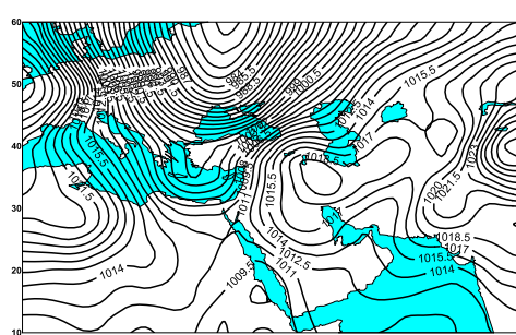
شکل ۳۵- میدان فشار (hpa) در ساعت ۰۰۰۰ گرینویچ ۱۸ ژانویه ۲۰۰۰.
