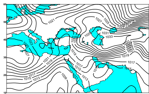
شکل ۷- میدان فشار (hpa) در ساعت ۰۰۰۰ گریجوی ۱۱ مارس ۲۰۱۵.
