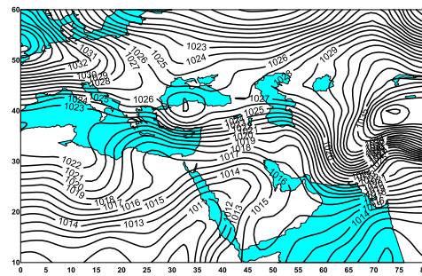
شکل ۲۹- میدان فشار (hpa) در ساعت ۰۰:۰۰ گرینویچ ۱۶ ژانویه ۲۰۰۰.
