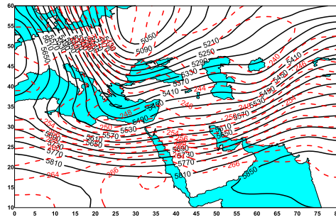
شکل ۳۷- میدان ارتفاع ژئوپتانسیل (gpm) و دما (k) در تراز ۵۰۰ هکتوپاسکال در ساعت ۰۰۰۰ گرینویچ ۱۸ ژانویه ۲۰۰۰.
