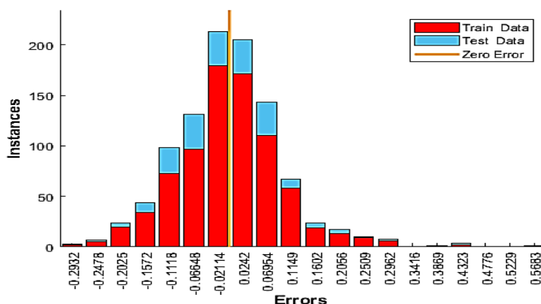
شکل ۷- هیستوگرام خطا به ازای داده‌های آموزشی و آزمایشی در شبکه عصبی پایه‌ای- شعاعی
