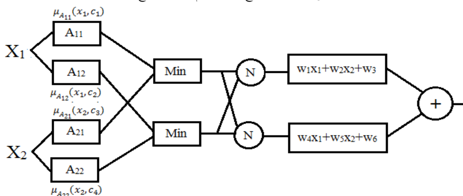
شکل ۳- ساختار سیستم استنتاج فازی - عصبی ANFIS
