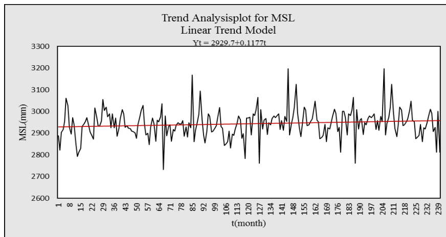
شکل ۸- نمودار روند تغییرات ماهانه میانگین تراز سطح دریا در ایستگاه چابهار
