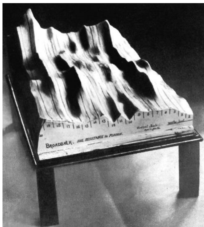
شکل ۲- مدل ۳ بعدی تغییرات مقاومت مکانیکی خاک (از Haines و Keen، ۱۹۲۵b)
