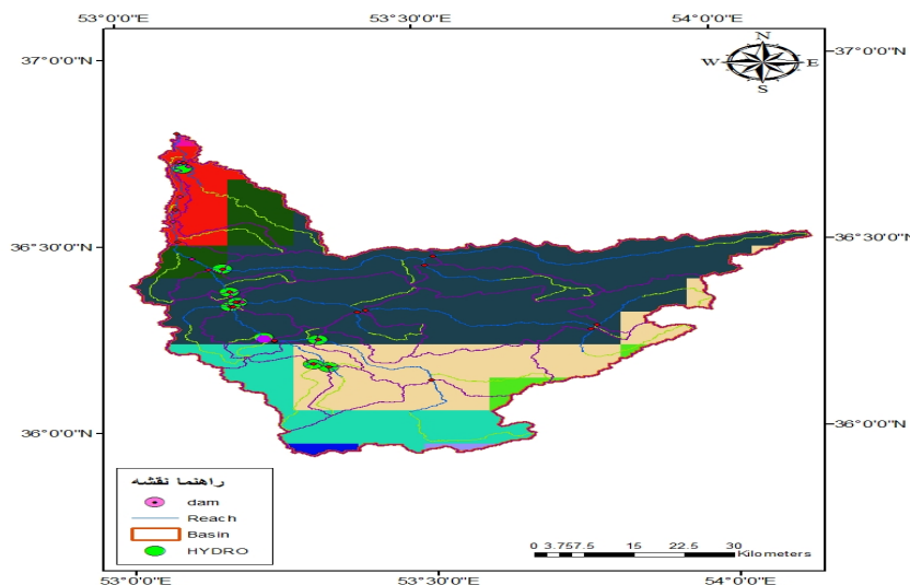
شکل ۱- موقعیت حوضه آبخیز تجن
