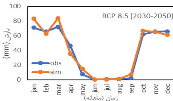
شکل ۴. ارزیابی شدت بارش و میزان آن تحت سناریوهای مختلف در ایستگاه سینوپتیک پل سفید
