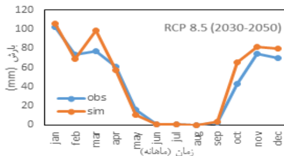
شکل ۶. ارزیابی شدت بارش و میزان آن تحت سناریوهای مختلف در ایستگاه باران‌سنجی نکا
