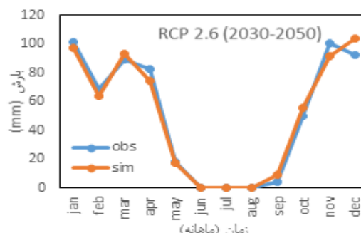
شکل ۷. ارزیابی شدت بارش و میزان آن تحت سناریوهای مختلف در ایستگاه باران‌سنجی داراب
