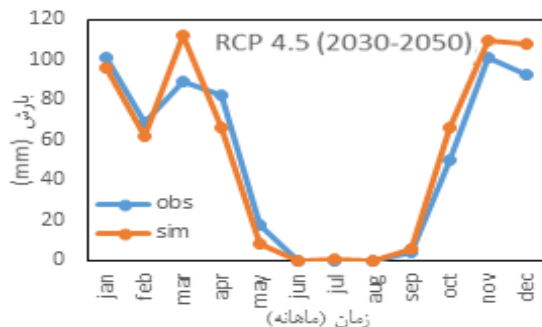
شکل ۷. ارزیابی شدت بارش و میزان آن تحت سناریوهای مختلف در ایستگاه باران‌سنجی داراب
