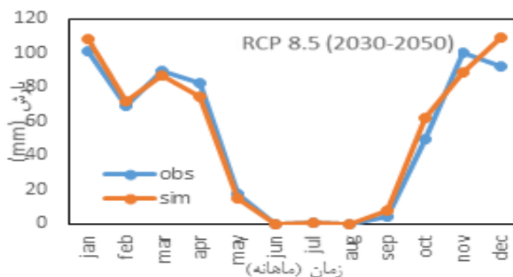
شکل ۸. ارزیابی شدت بارش و میزان آن تحت سناریوهای مختلف در ایستگاه باران‌سنجی کیاسر
