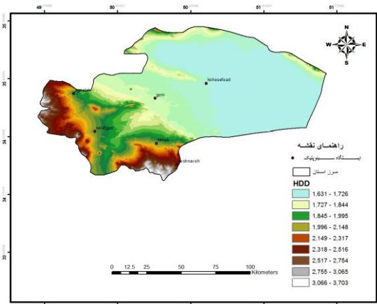
شکل ۸- مجموع سالانه نیاز گرمایشی (راست) و سرمایشی (چپ) محیط گلخانه کشت سبزیجات پر مصرف در استان قم
