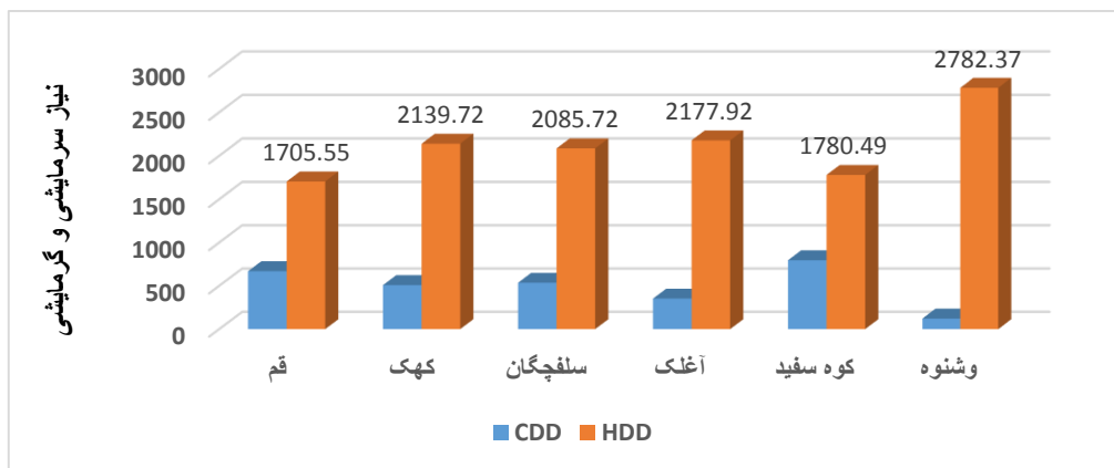
نمودار (۱) مجموع سالانه نیاز گرمایشی و سرمایشی محیط گلخانه در ایستگاه‌های منتخب استان قم
