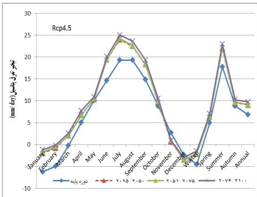
شکل ۵- تغییرات میانگین ماهانه تبخیر- تعرق پتانسیل میانگین دو مدل CMIP5 (۱.۱) BCC-CSM و CCSM4) تحت سناریوی RCP 4.5
