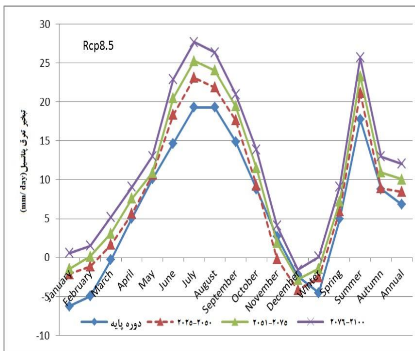
شکل ۶- تغییرات میانگین ماهانه تبخیر- تعرق پتانسیل میانگین دو مدل CMIP5 (۱.۱) BCC-CSM و CCSM4) تحت سناریوی RCP 8.5
